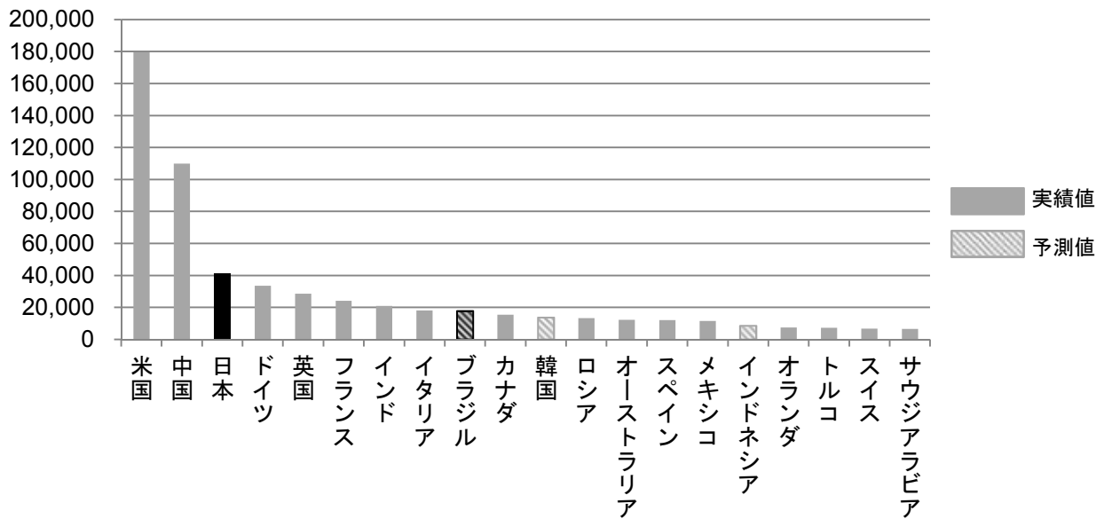
名目GDP (2015年)
